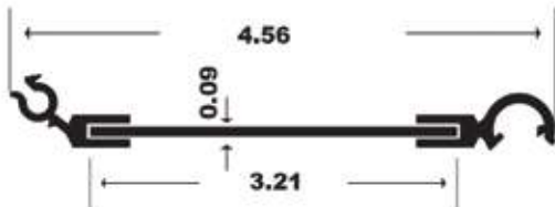
313 - CLEAR BLADE
