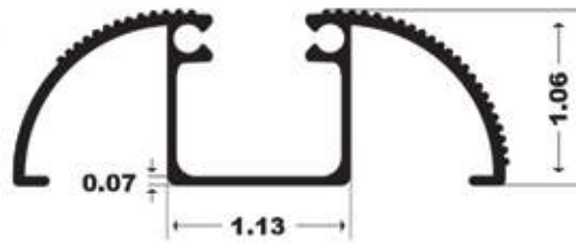
359 - WALKOVER
