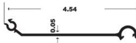
371 - BLADE
